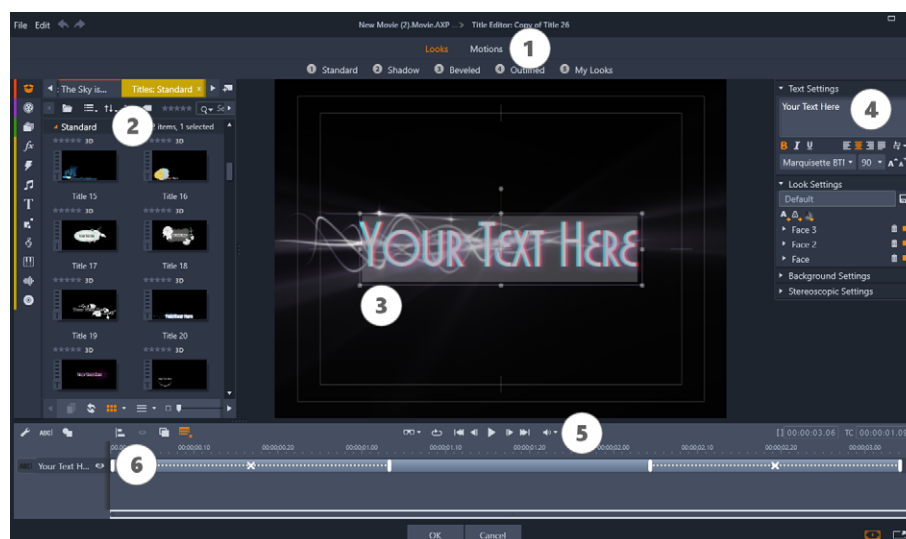
Obszary Edytora tytułu: 1. Moduł wyboru ustawień wstępnych; 2. Panel Biblioteka; 3. Okno edycji; 4. Panel Ustawienia; 5. Pasek narzędzi; 6. Lista warstw
